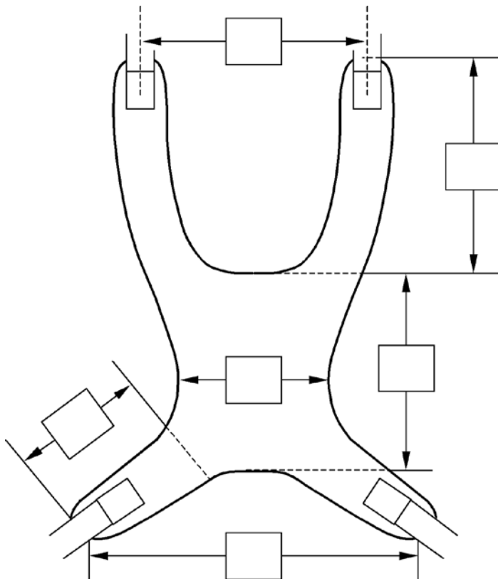
Brustschulterpelotte
